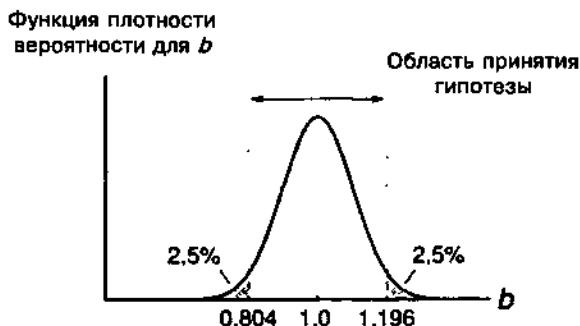
Рис. 3.6. Область принятия гипотезы для величины b при 5-процентном уровне значимости
