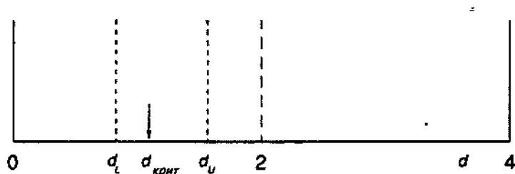
Рис. 7.5. Тест Дарбина—Уотсона на автокорреляцию (показана зона неопределенности в случае предполагаемой положительной автокорреляции)
