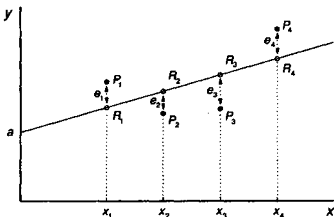
Рис. 2.3. Построенная по точкам линия регрессии, показывающая остатки
