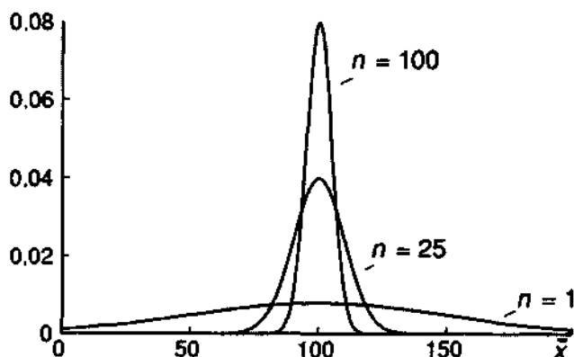
Рис. 0.11. Влияние увеличения размера выборки на распределение \bar{x} .
