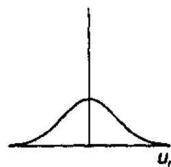
Рис. 7.1. Различия между гетероскедастичностью и гомоскедастичностью
