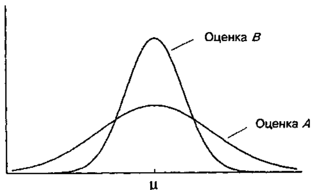
Рис. 0.8. Эффективные и неэффективные оценки
