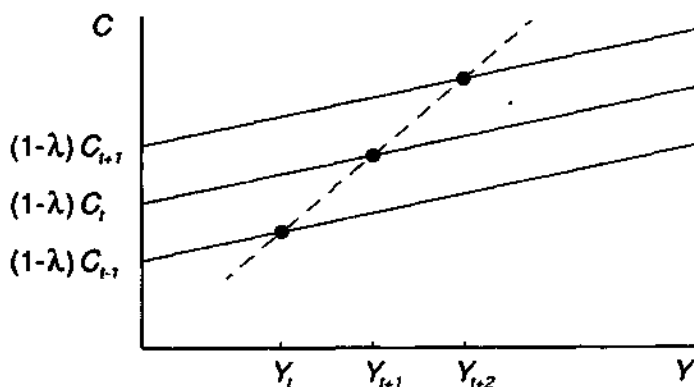
Рис. 10.1. Динамические свойства модели постоянного дохода Фридмана
