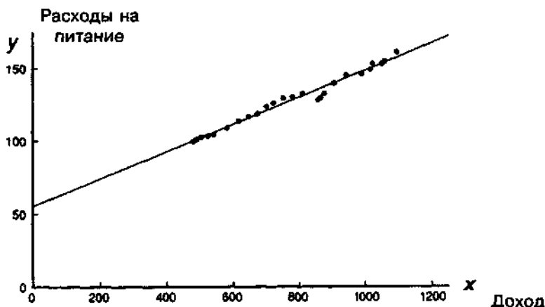
Рис. 2.7. Регрессионная зависимость расходов на питание от доходов (США, 1959–1983 гг.)
